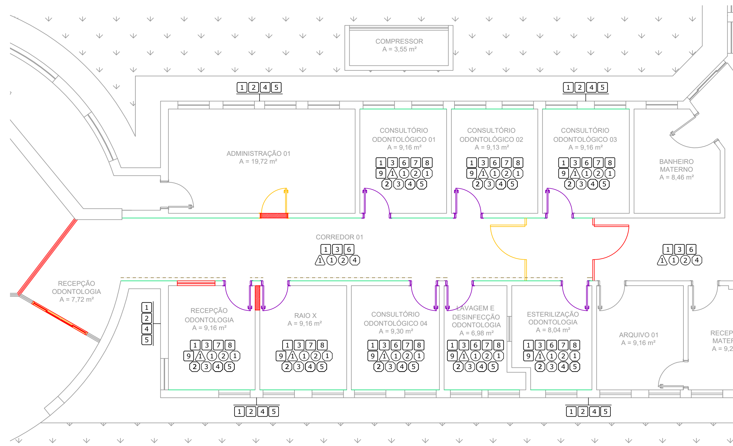
PLANTA BAIXA - CEO Escala: 1:75
