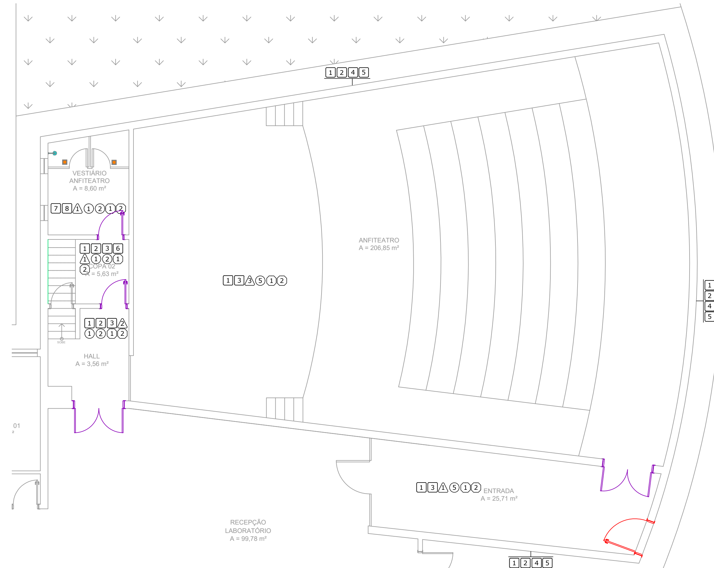
PLANTA BAIXA - ANFITEATRO Escala: 1:75
